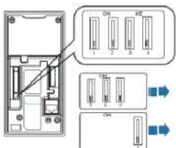
Согласующее сопротивление (DIP4)
