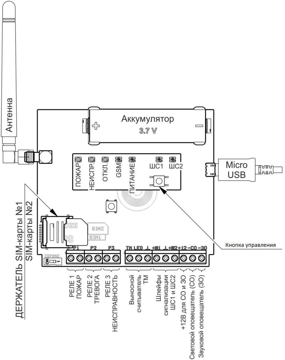
Рис.9. Вид платы прибора
