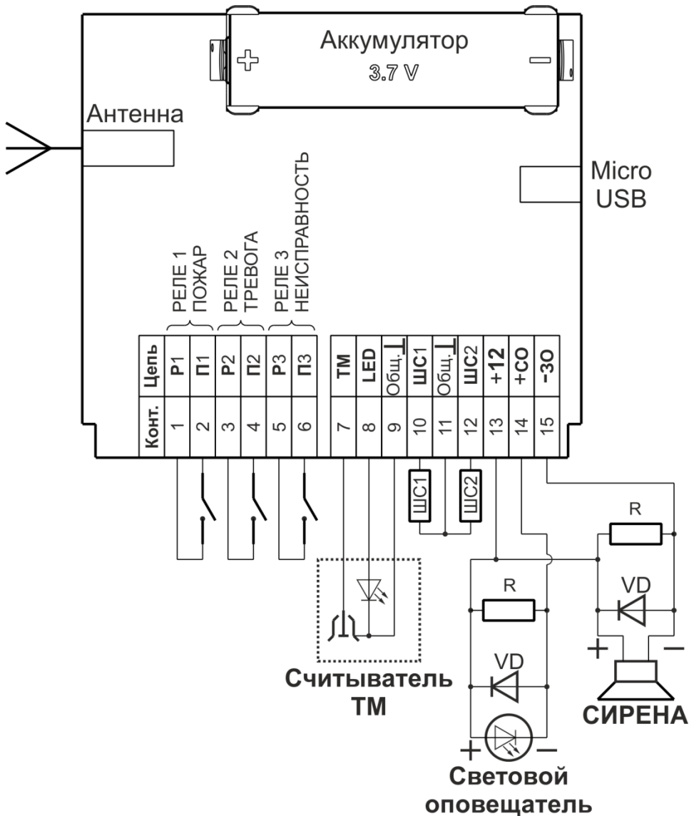
Рис.4. Схемы внешних соединений прибора
