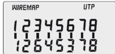
Результат при перекрещивании линий «3» и «6» кабеля RJ45
