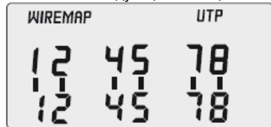
Результат при обрыве линий «3» и «6» кабеля RJ45
