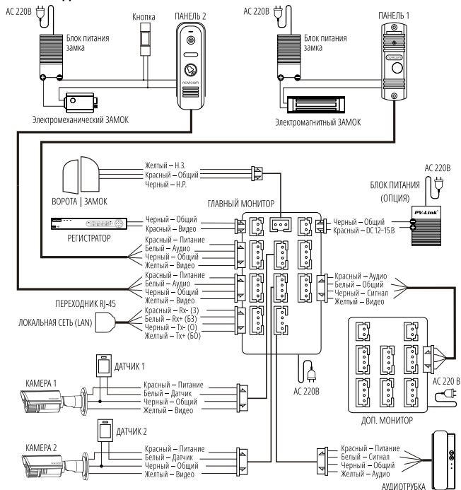
Рис. 9 Схема подключения видеодомофонов FREEDOM
