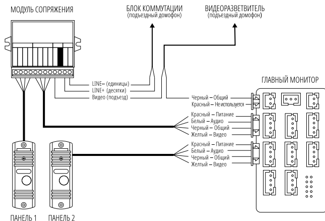
Рис. 11 Подключение монитора FREEDOM к подъездному домофону через модуль сопряжения
