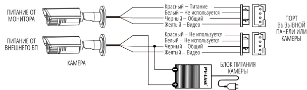
Рис. 10 Схемы подключения видеокамеры к монитору FREEDOM
