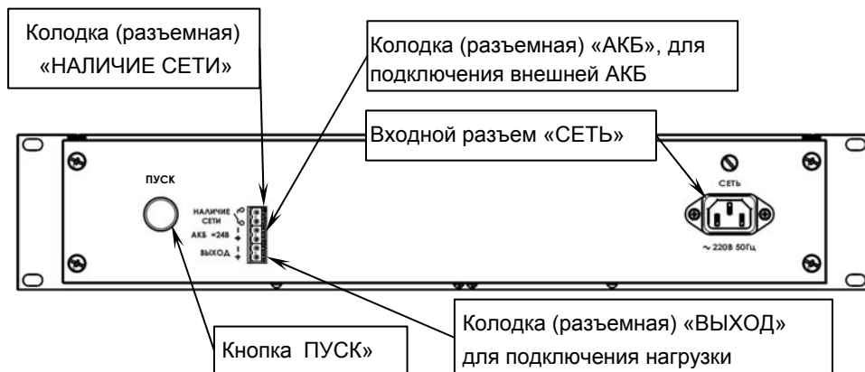
Рисунок 2 – задняя панель изделия
