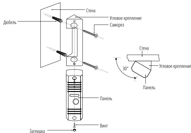
Рис. 8 Установка вызывной панели под углом 30°
