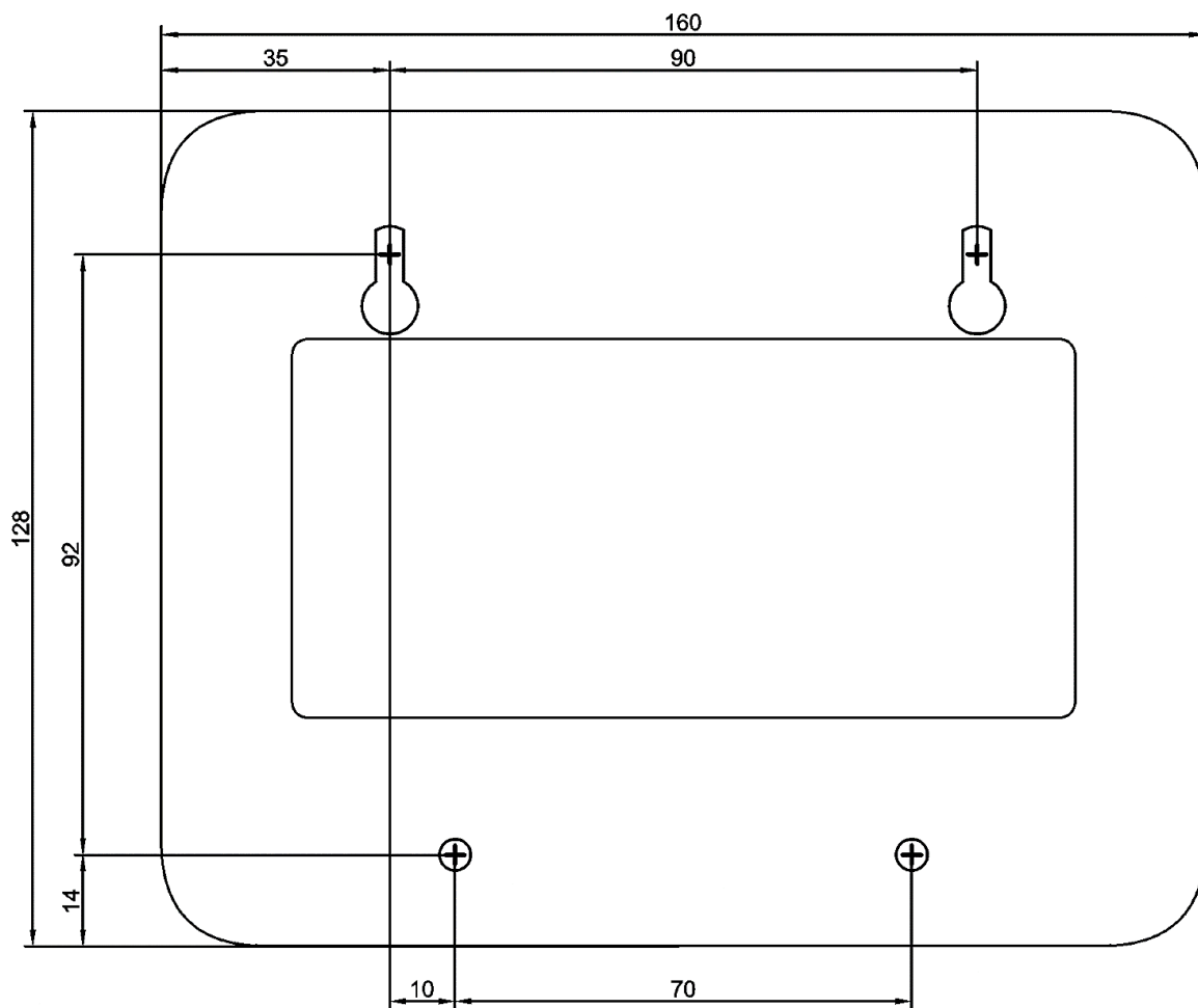
Рисунок Л.4 - Разметка отверстий для крепления прибора КОП-02.4 (вид со стороны передней панели)
