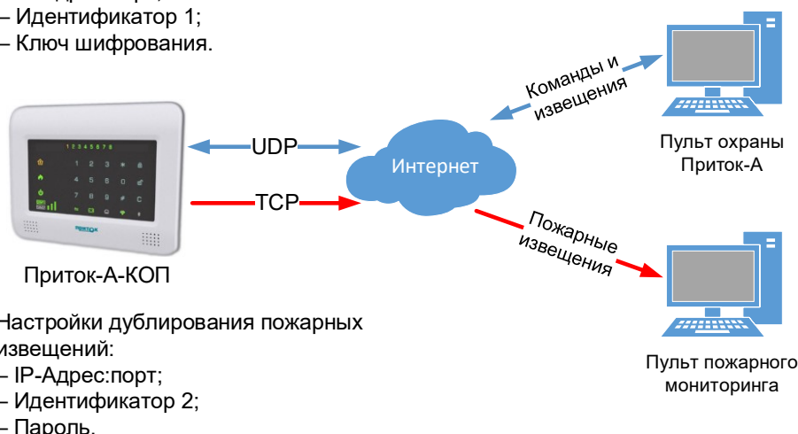
Рисунок 2.21.1 – Схема работы прибора с пультом пожарного мониторинга
