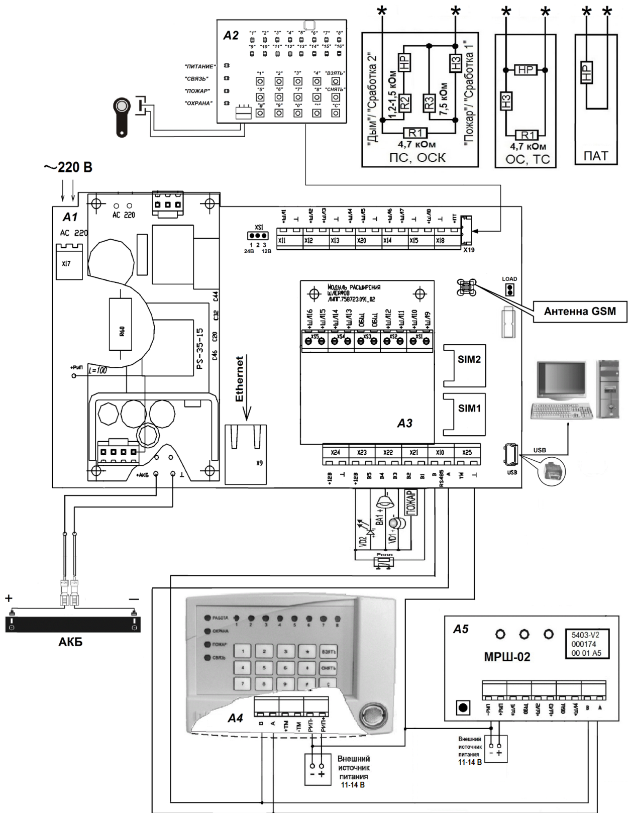
Рисунок А.1 – Схема подключения прибора версии Приток-А-КОП-01
