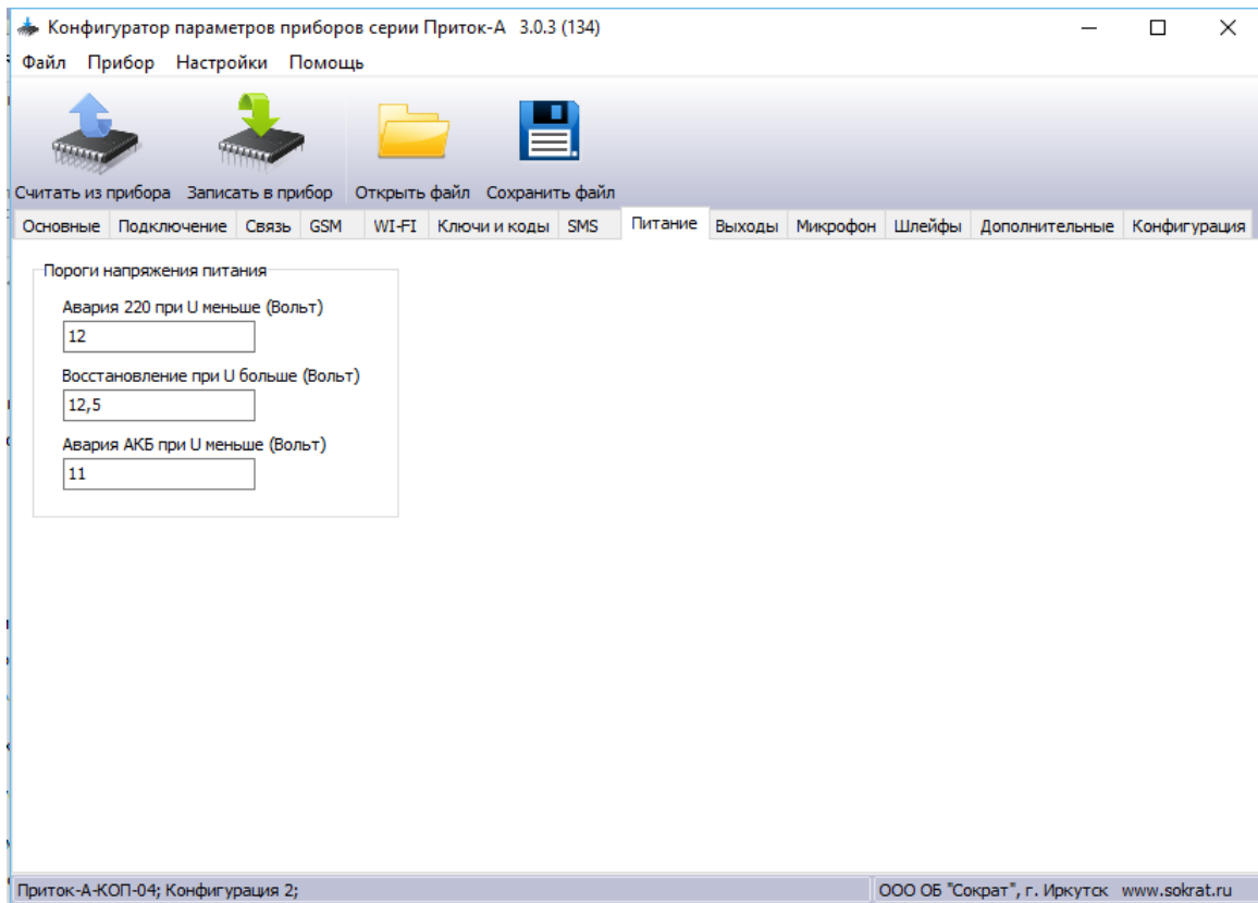
Рисунок 2.14 - Вкладка «Питание»
