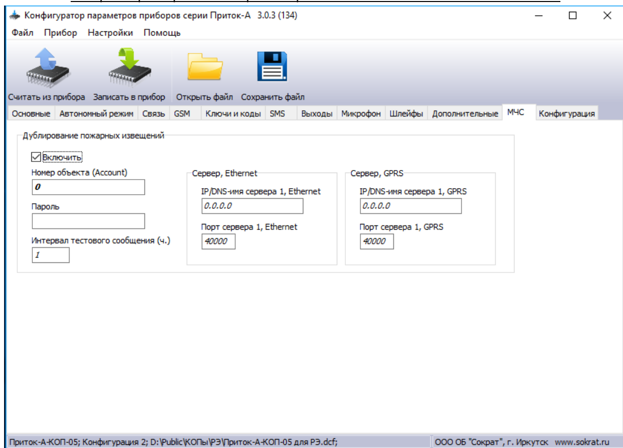
Рисунок 2.21 – Вкладка «МЧС»
