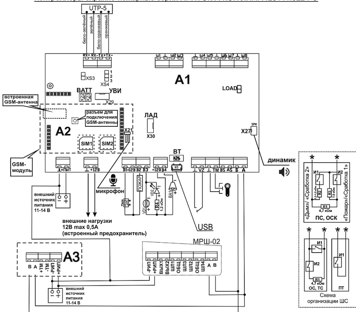
Рисунок А.12 - Схема подключения прибора версии Приток-А-КОП-04 (D)
