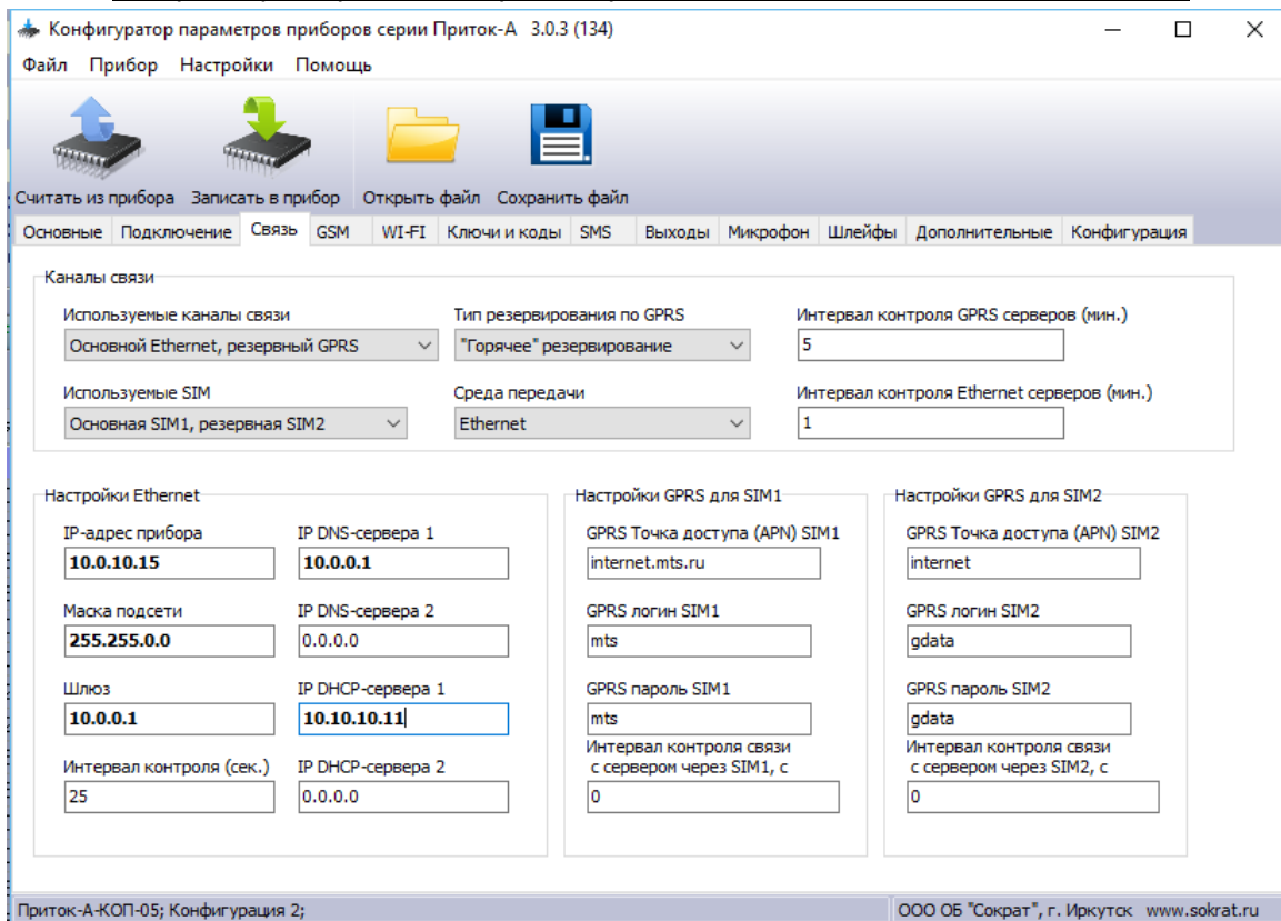
Рисунок 2.8 - Вкладка «Связь»
