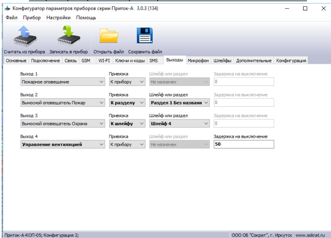
Рисунок 2.15 - Вкладка «Выходы»
