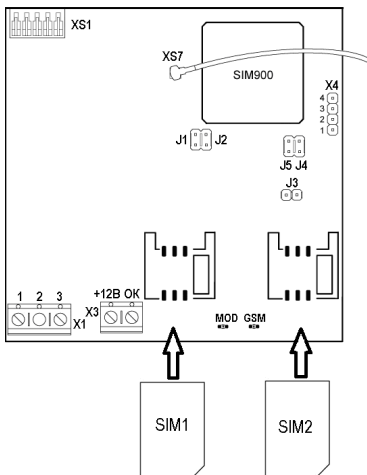
Рисунок 15.1 – Коммуникатор
