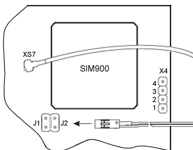
Рисунок 15.4 – Подключение термодатчика
