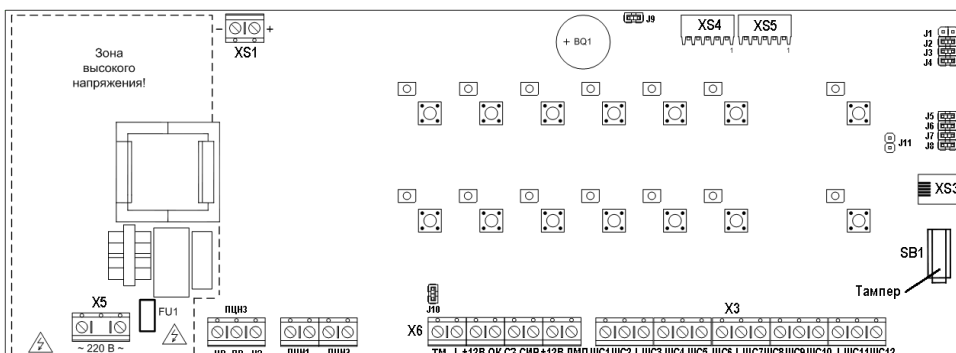
Рисунок 4.1 – Внешний вид платы прибора
