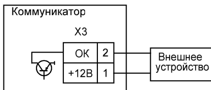
Рисунок 15.2 – Схема подключения внешнего устройства к коммуникатору
