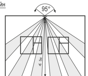
Г) Вариант установки на потолке
