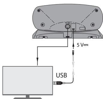
Питание от ТВ
