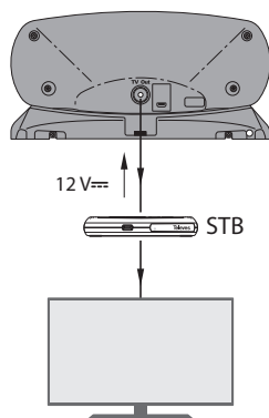
Питание от приемника (B4 коннектор)
