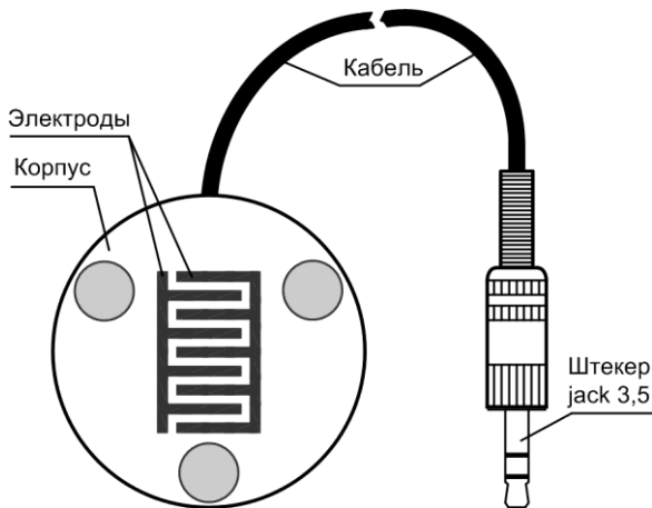
Рис.3 Датчик протечки воды
