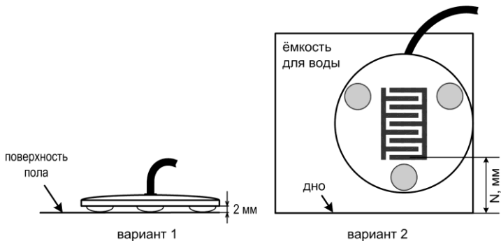
Рис.9 Примеры расположения датчика протечки воды
