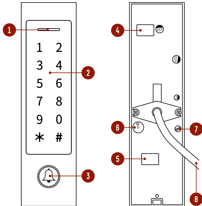
Рис. 2 Описание контроллера SE410KW WIFI
