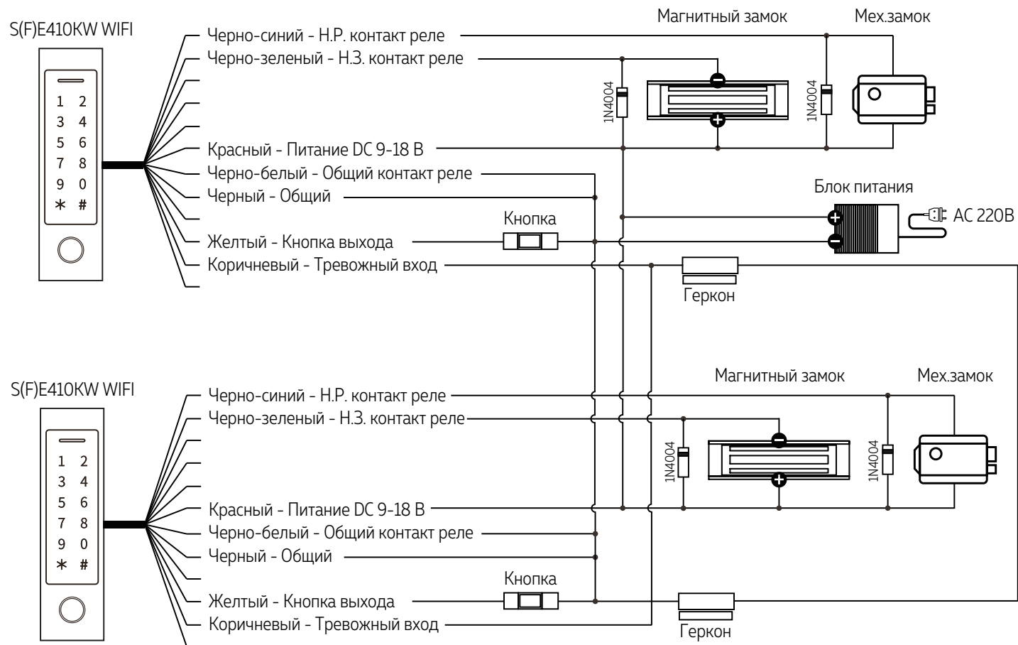
Рис. 9 Схема подключения контроллеров для организации шлюза
