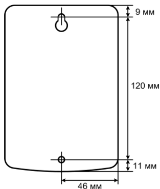
Рис.5б Основание сирены. Положение отверстий для крепежа. Присоединительные размеры
