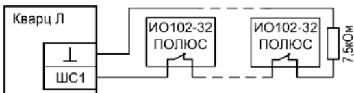
Рис.А4 Схема подключения магнитоконтактных охранных извещателей ПОЛЮС
