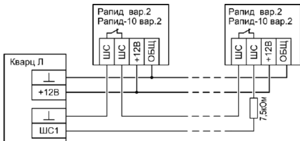
Рис.А7 Схема подключения охранных извещателей Рапид вар.2, Рапид-10 вар.2
