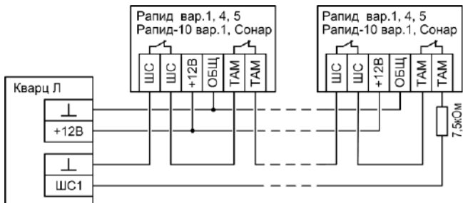
Рис.А6 Схема подключения охранных извещателей Рапид вар.1, 4, 5, Рапид-10 вар.1 и Сонар
