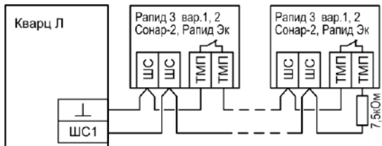
Рис.А5 Схема подключения охранных извещателей с питанием по ШС
